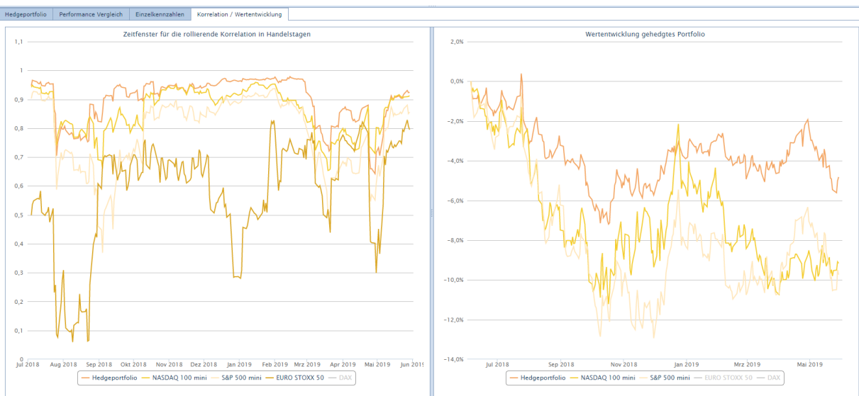
Abbildung 2: Korrelation und Wertentwicklung kombiniert
